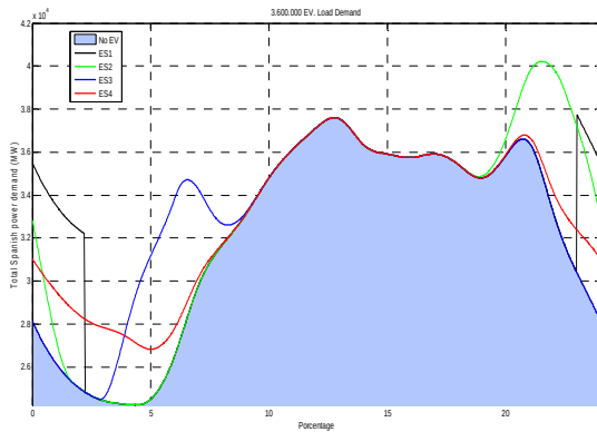
Fig.9. Total load demand NoEV-ES1-ES2-ES3-ES4 (2017)
