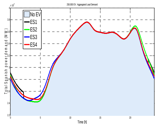
Fig.7. Total load demand NoEV-ES1-ES2-ES3-ES4 (2014)
